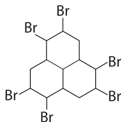
Figure 1 : Formule développée du HBCD
