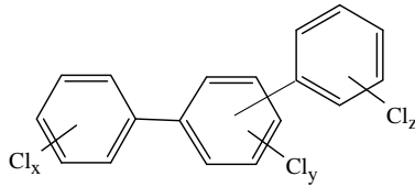
图 2：多氯三联苯的化学结构图
