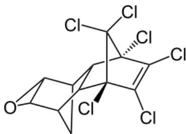
Figure 4 : Formule structurelle de la dieldrine
