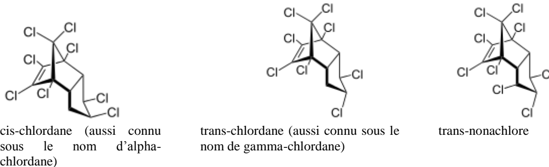
Figure 2 : Formules structurelles des composants du chlordane
