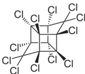
Figure 10 : Formule structurelle du mirex
