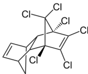
Figure 1 : Formule structurelle de l'aldrine
