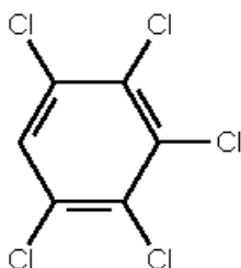
Figure 11 : Formule structurelle du pentachlorobenzène
