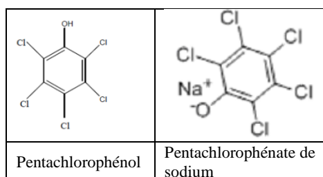
Figure 10 : Formules structurales du PCP et de son sel de sodium
