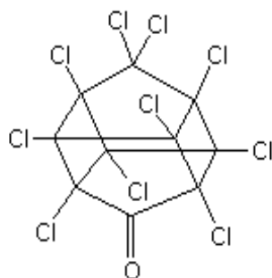
Figure 3 : Formule structurelle du chlordécone
