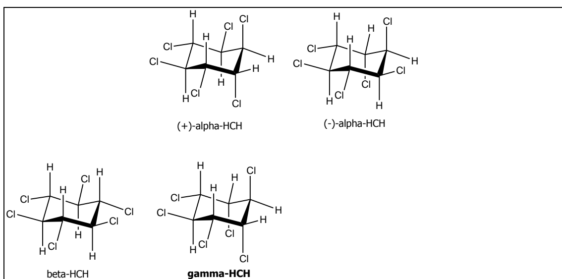
Figure 9 : Formules structurales du lindane (gamma-HCH), de l'alpha-HCH et du bêta-HCH
