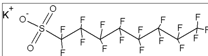
Figure 13 : Formule structurelle du SPFO
