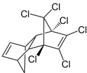
Рисунок 1: Структурная формула альтрина
