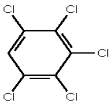
Рисунок 11: Структурная формула пентахлорбензола
