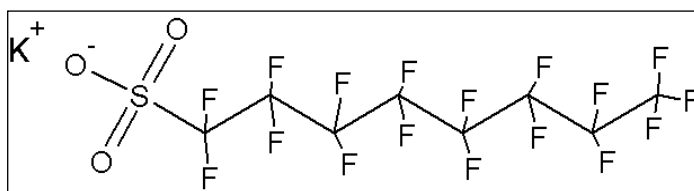
Рисунок 13: Структурная формула ПФОС
