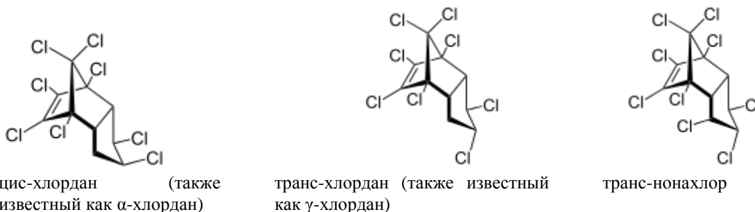
Рисунок 2: Структурная формула компонентов хлордана
